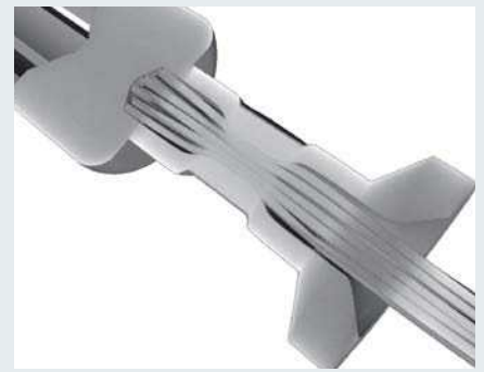
Ansicht längs durch den Crimp
