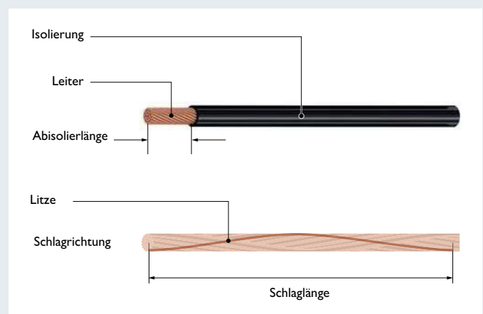
Standardleitersaufbau
