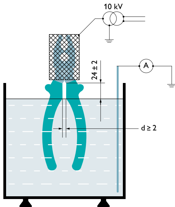
Vorrichtung zur Spannungsprüfung isolierter Handwerkzeuge (DIN EN 60900 Bild 15)
