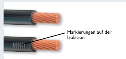
Einwandfrei abisolierte Leiter nach DIN IEC 60352-2
