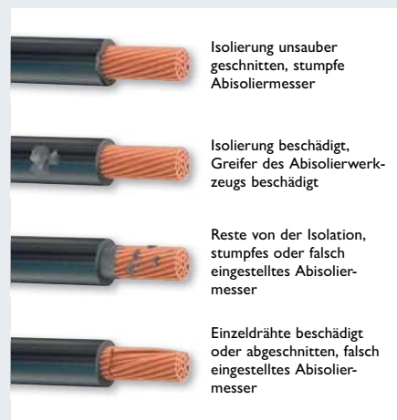
Abisolierfehler nach DIN IEC 60352-2
