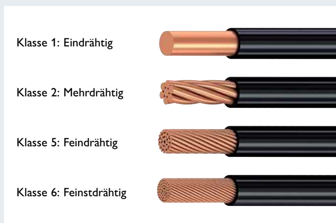
Leiterklassen nach IEC/DIN EN 60228 (VDE 0295)
