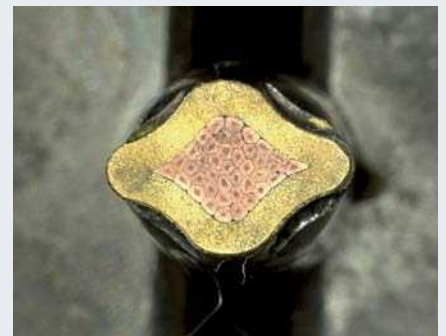
Schliffbild
